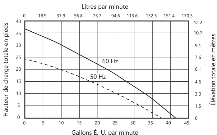
Figure 3. Rendement hydraulique de l'appareil
